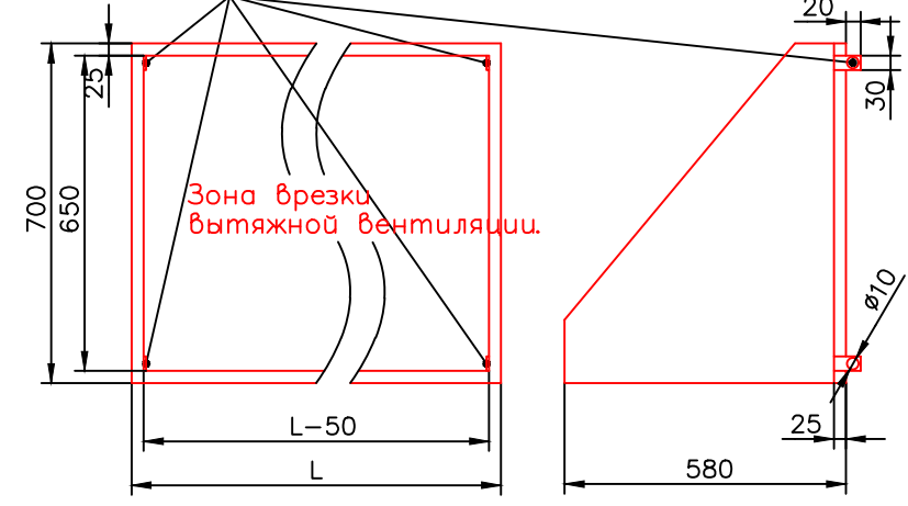
МВО-МСВ Скобы для подвески
