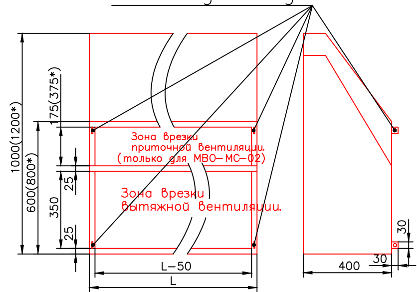
МВО-МС Скобы для подвески
