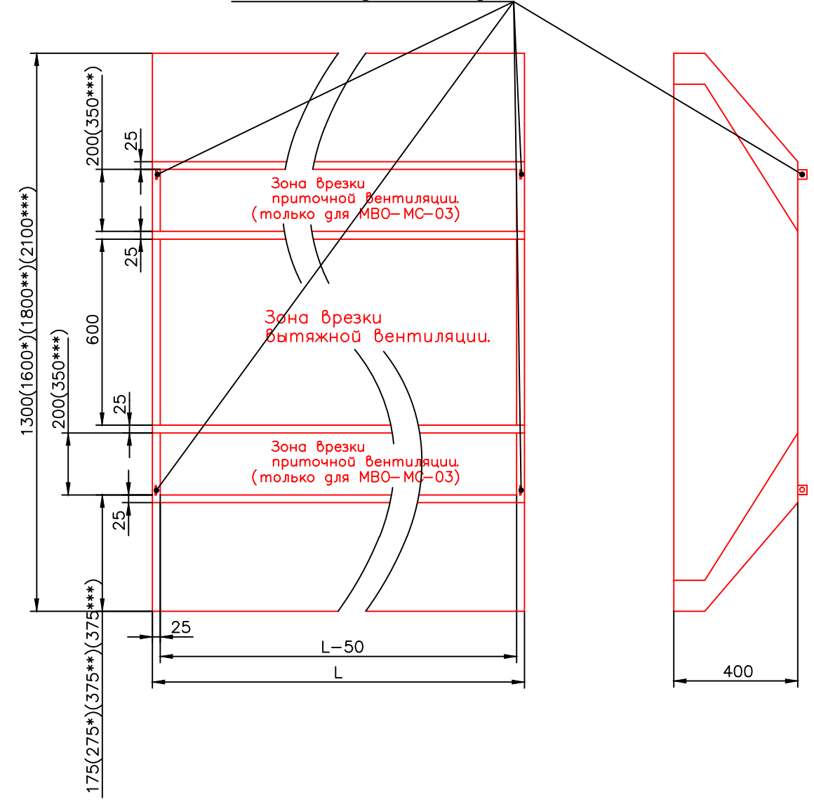
МВО-МС(МСВ)-03x1,3(1,6*)(1,8**)(2,1***) Скобы для подвески
