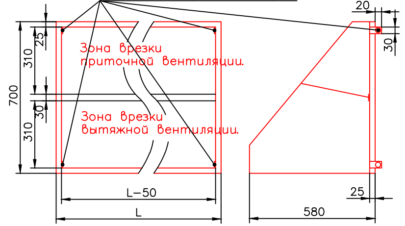
МВО-МС Скобы для подвески
